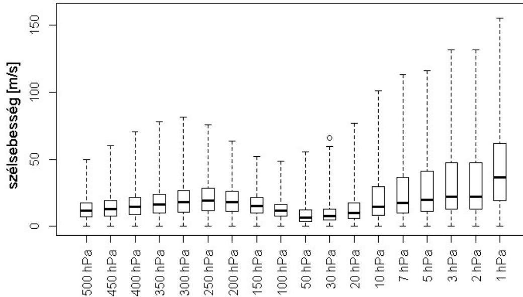
2. ábra: A szélességek eloszlása a vizsgált szinteken 500 hPa – 1 hPa szintig az 1979–2015 időszak adatai alapján. A dobozok alsó és felső lapja jelöli az alsó és felső kvartilis értéket, a dobozokban lévő vastagabb vízszintes vonal az adott nyomási szint szélességeinek medián értékeit, míg a szaggatott függőleges vonal alsó és felső vége a legkisebb és legnagyobb szélesség értékeit.
