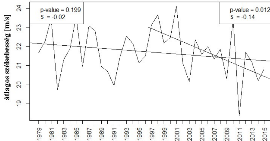
7. ábra: Az éves átlagos szélességek trendje a 250 hPa nyomási szinten a kivágtat összes rácspontját számításba véve (1979–2015).
