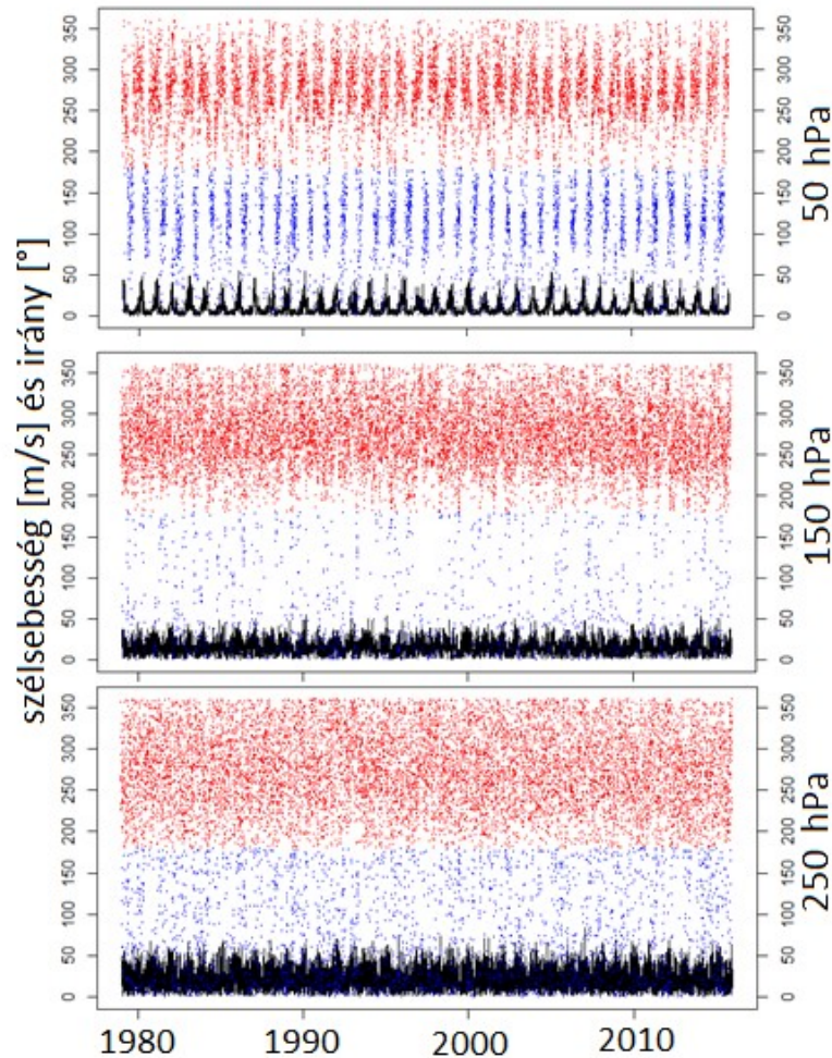
6. ábra: A szélességek (fekete vonal) és irányok (keleties - kék, nyugatias - piros) idősora a Budapesthez legközelebb eső rácspontban (É.sz. 47,25°, K.h. 18,75°) az 1979–2015 időszakra.
