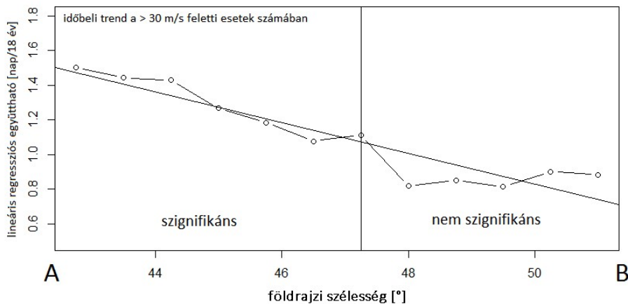
8. ábra: A lineáris regressziós együttható értékek a 30 m/s feletti szélességek éves esetszám idősorára a k.h. 18.75° hosszúsági kör mentén (1997–2015).
