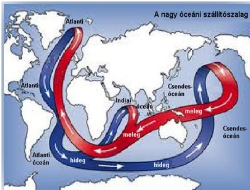
9. ábra: A nagy óceáni szállítószalag. Piros színnel a meleg felszíni, míg kék színnel a hideg mélyóceáni áramlatokat jelöljük (az Egyenlítő felé haladó felszíni áramlatok a környezetüknél hidegebb, míg az alacsonyabb szélességek felé tartó áramlatok a környezetüknél melegebb víztömeget szállítanak) (Broecker (2010) és Weidinger & Tasnádi (2015) alapján).
