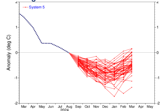
Tengerfelszín-hőmérséklet anomália
